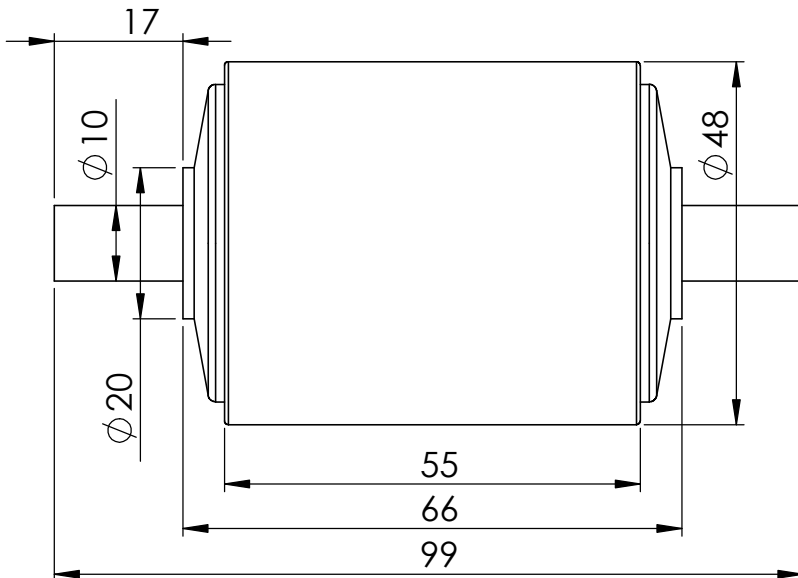
Walze mit Achse 1:1
